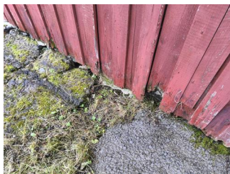
Veggkonstruksjon og fasadematerialer - Råteskade i kledning
