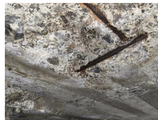
Fundament, grunnmur og gulv mot grunn - Eksponert armering med rust
