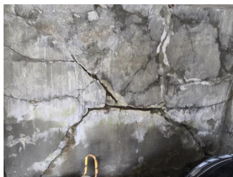
Fundament, grunnmur og gulv mot grunn - Betydelige skader i grunnmur og jordtryksskade
