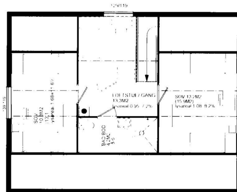
2.ET.PLAN
