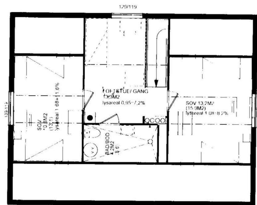
2.ET.PLAN
