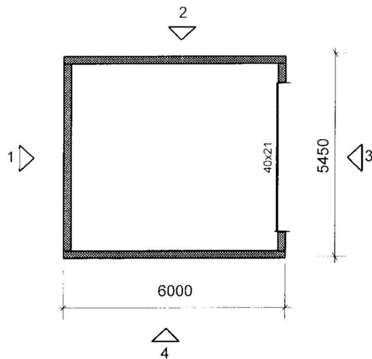
PLAN GARASJE
