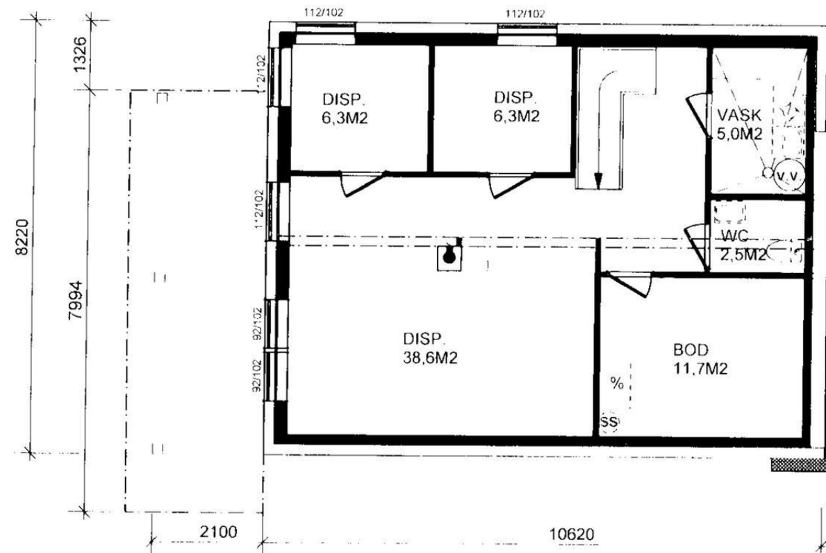
SOKKELPLAN
