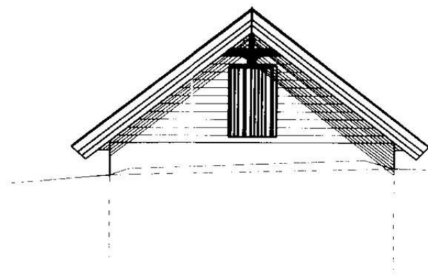
FASADE 1 mot sørøst
