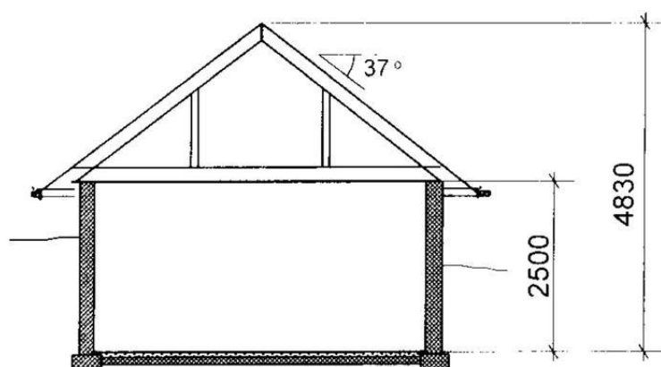
SNITT
