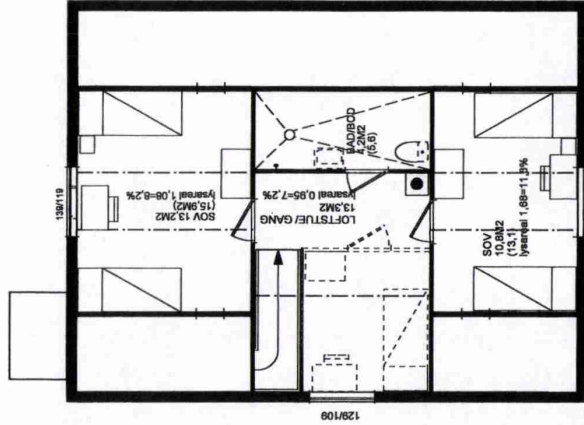
2. ET.PLAN
