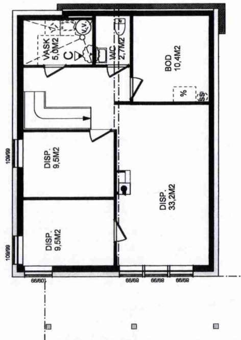
KJELLERPLAN
