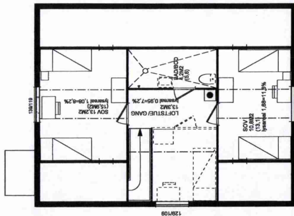
2. ET. PLAN
