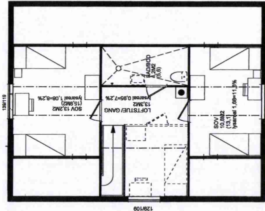
2.ET.PLAN
