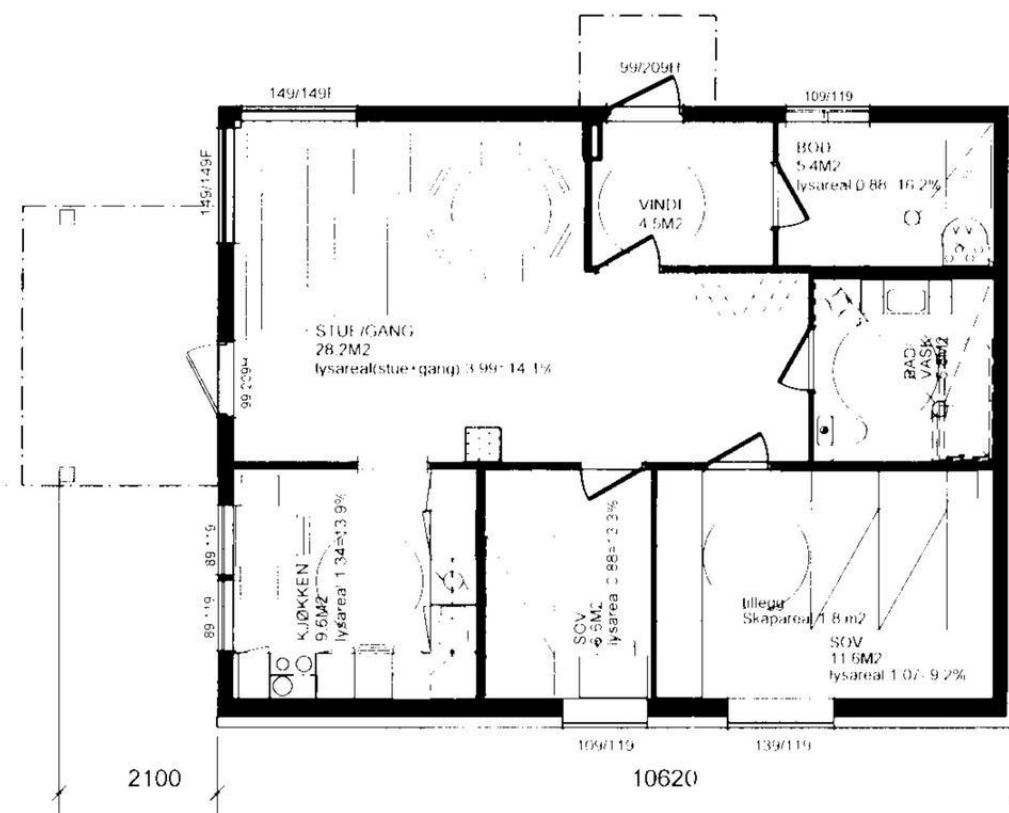
2.ET.PLAN
