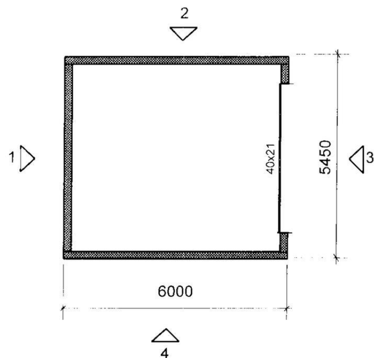
PLAN GARASJE
