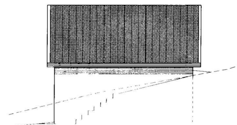
FASADE 2 mot sør
