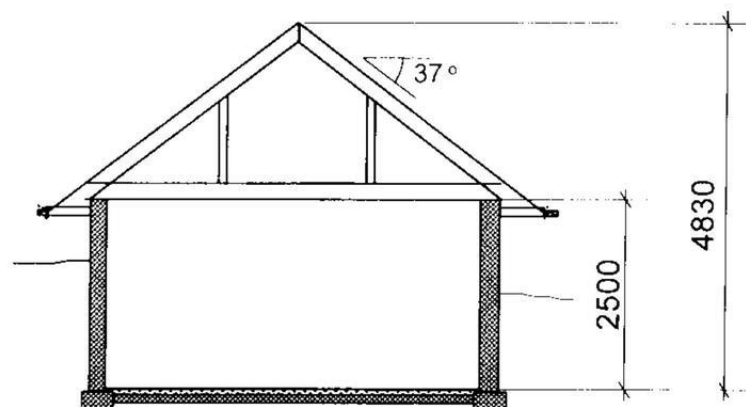
SNITT
