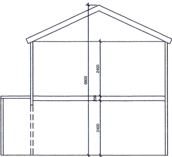
Snitt
