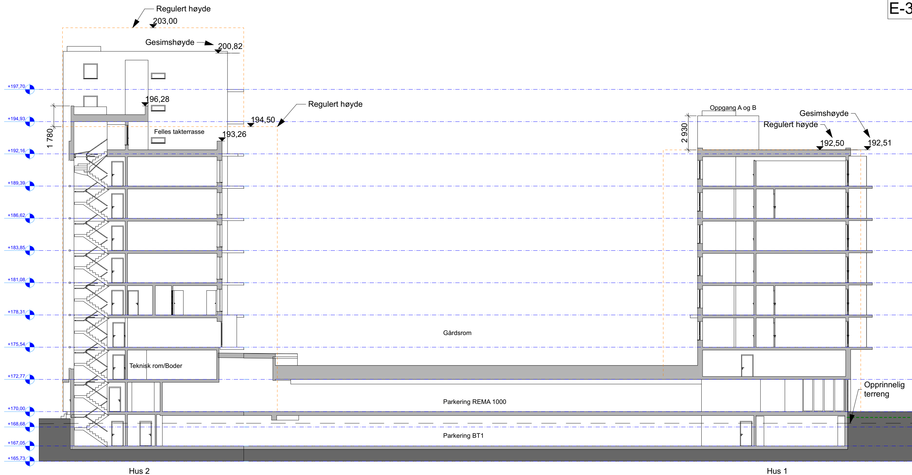
1:200 Schnitt B
