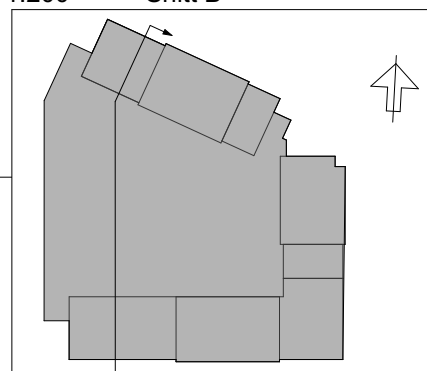
1:200 Schnitt B
