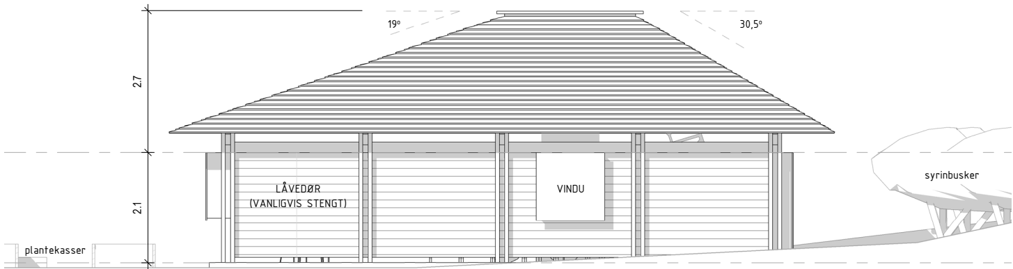
Østfasade
