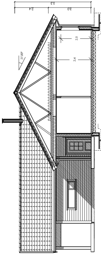
SNITT A-A
