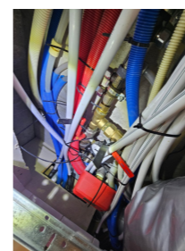
Vann rør montert i taket uten vannskap.
