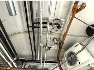
Rørføring under dekke for leiligheter.
