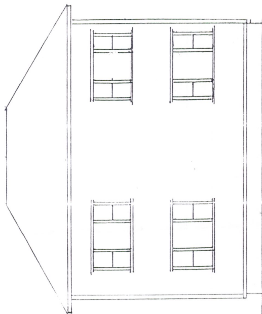
FASADE VEST
