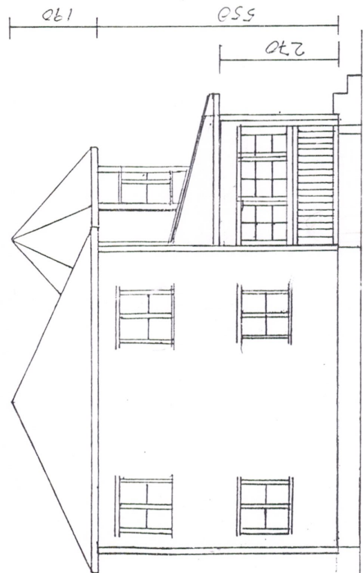
FASADE SYD
