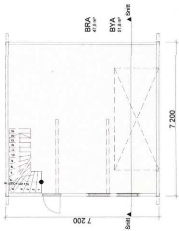
Plan 1 etasje 1:100
