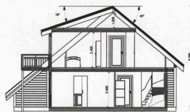
SNITT A-A
