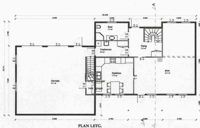
PLAN 1.ETG.
