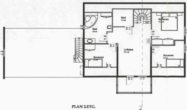
PLAN 2.ETG.
