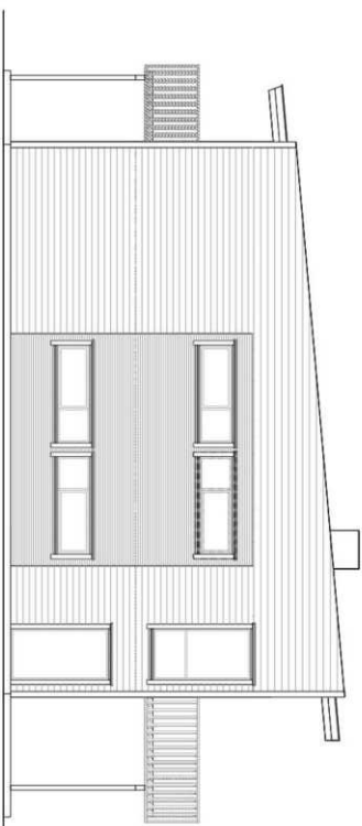
FASADE 4
