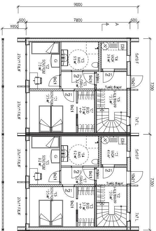
1. ETASJE
