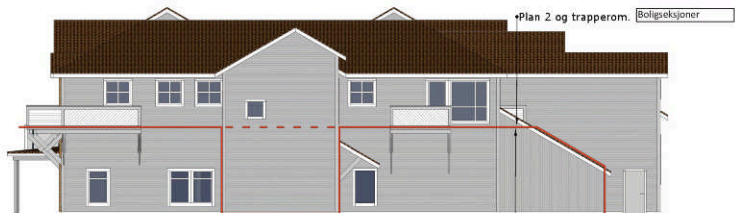
FASADE SYD
