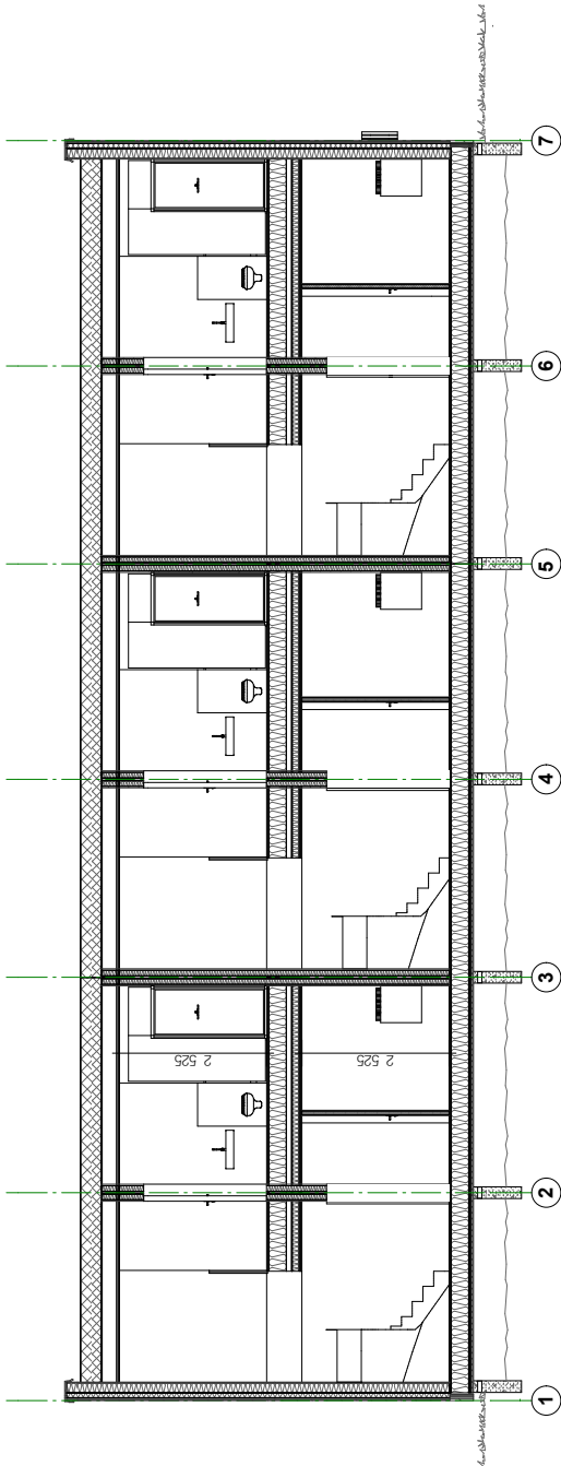
Snitt E-E
