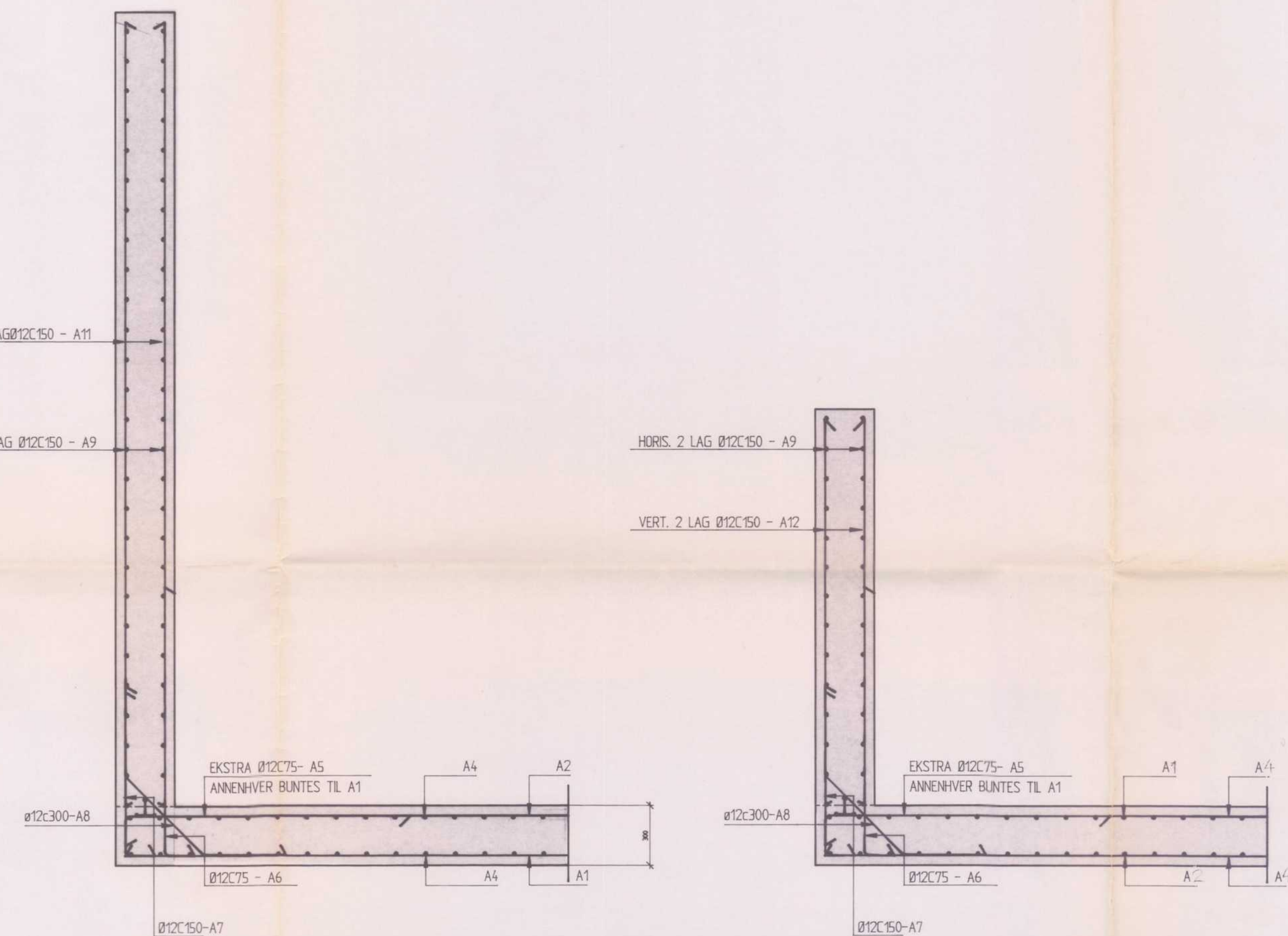
SNITT B-B
