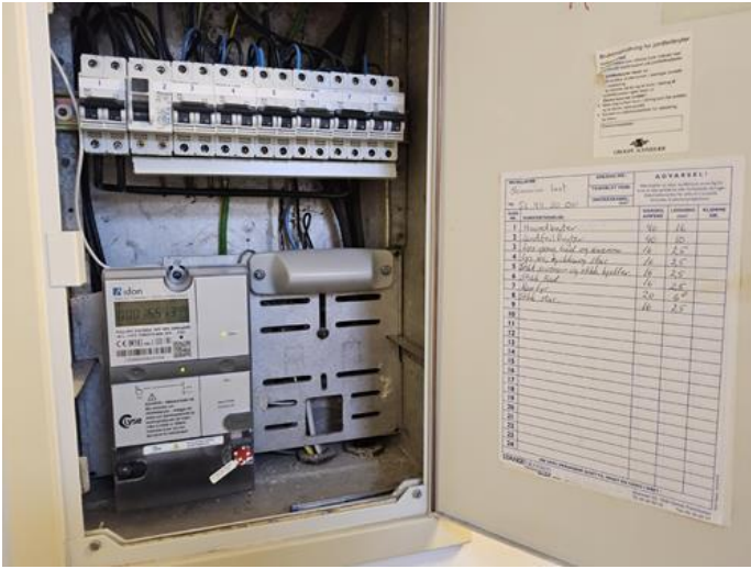
Elektrisk anlegg - [El-skap.]
