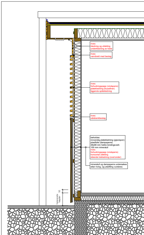
Veggsnitt 2 mot øst - eksisterende situasjon
