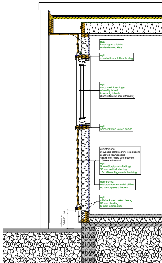
Veggsnitt 1 mot øst - etter fasadefornyning
