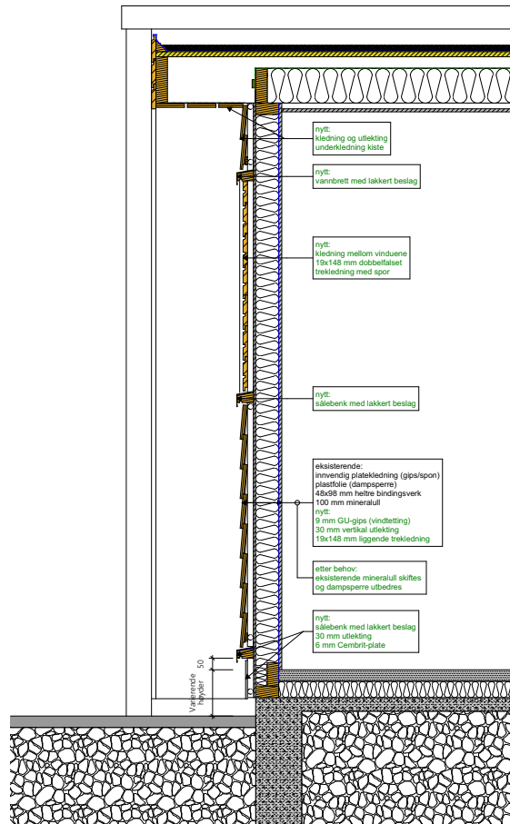
Veggsnitt 2 mot øst - etter fasadefornying
