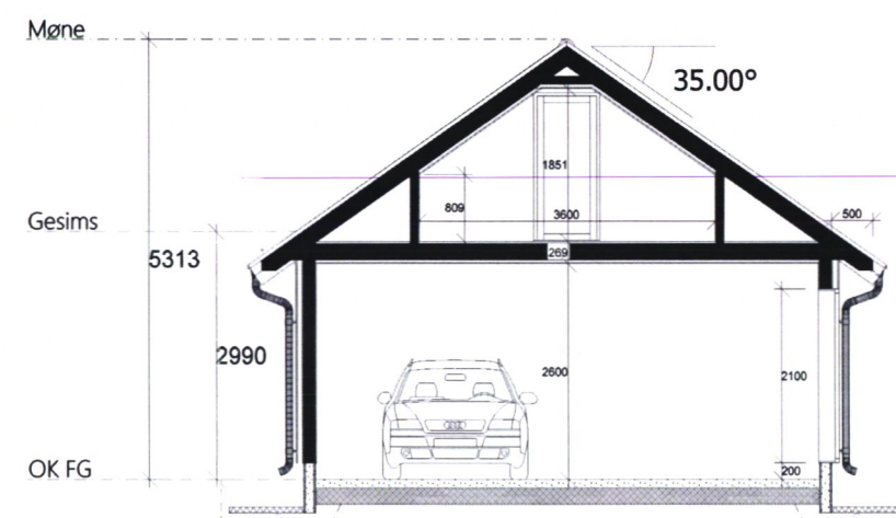
Snitt AA
