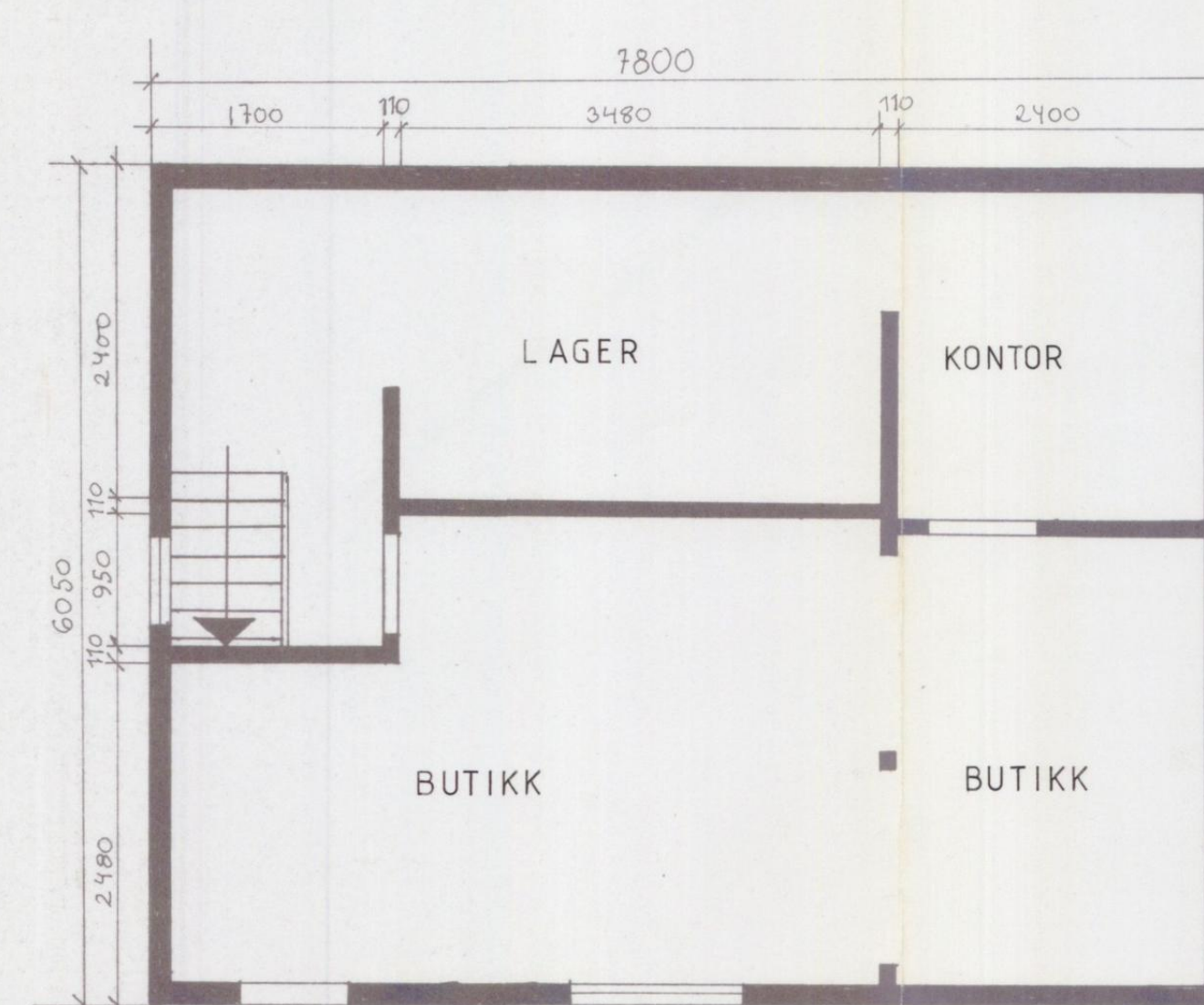
PLAN 1. ETG.
