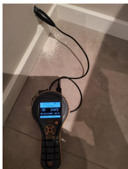
Kontroll i lukkede konstruksjoner - Relativ luftfuktighet.
