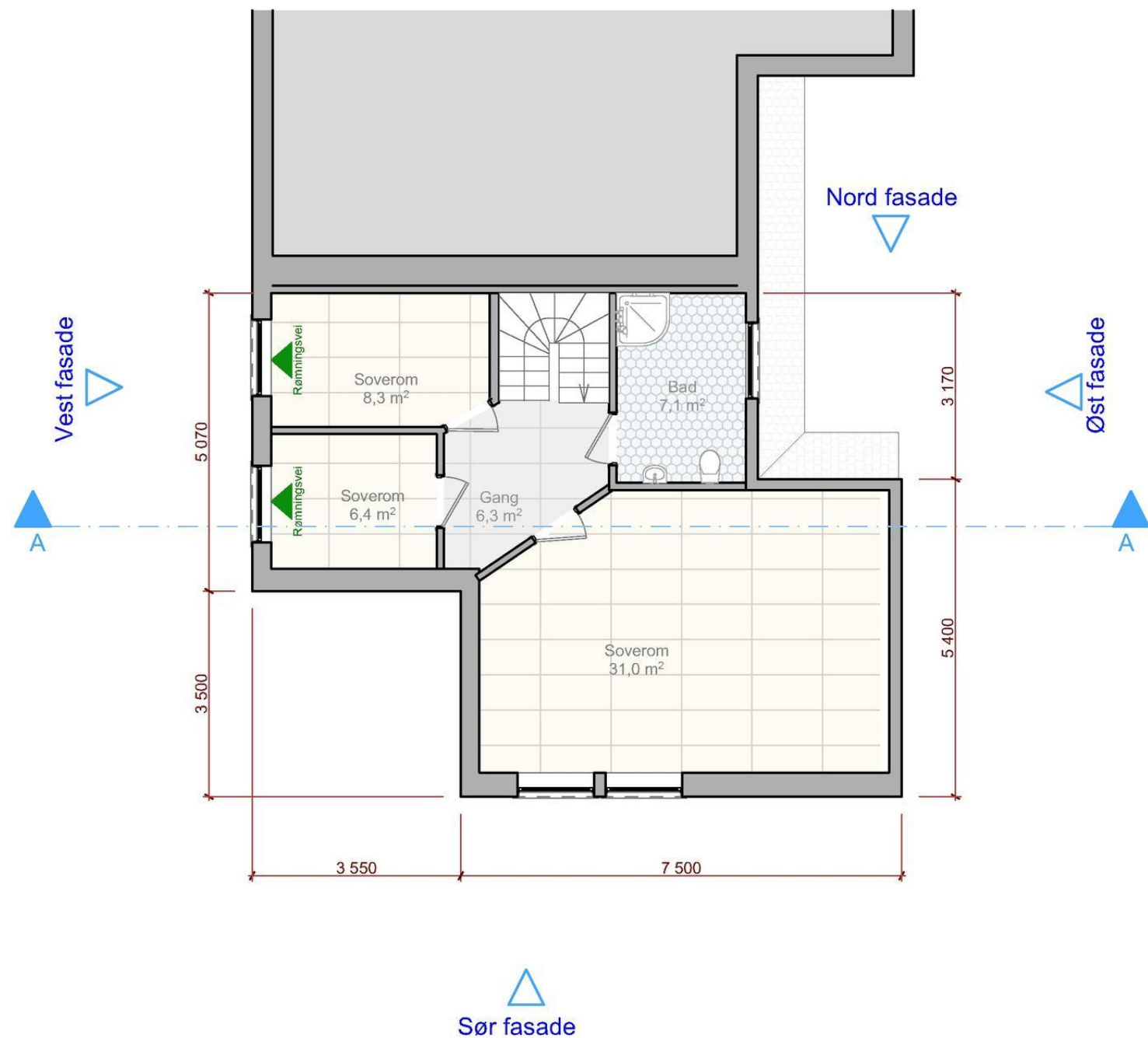
2 Etasje plan - Søkes om endringer
