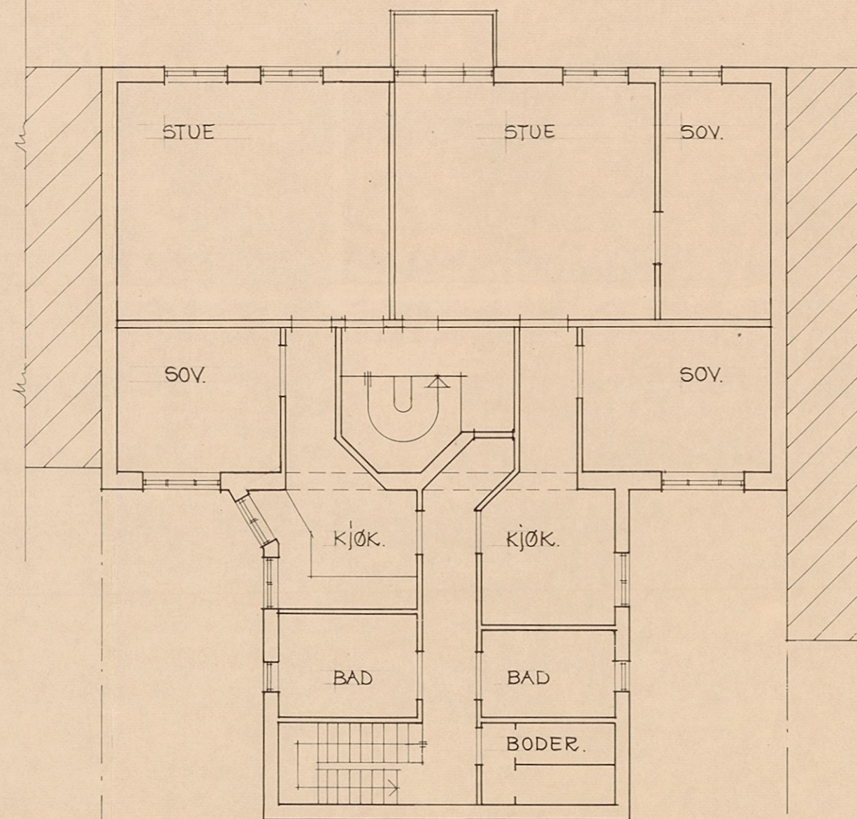
PLAN 4. ETASJE
