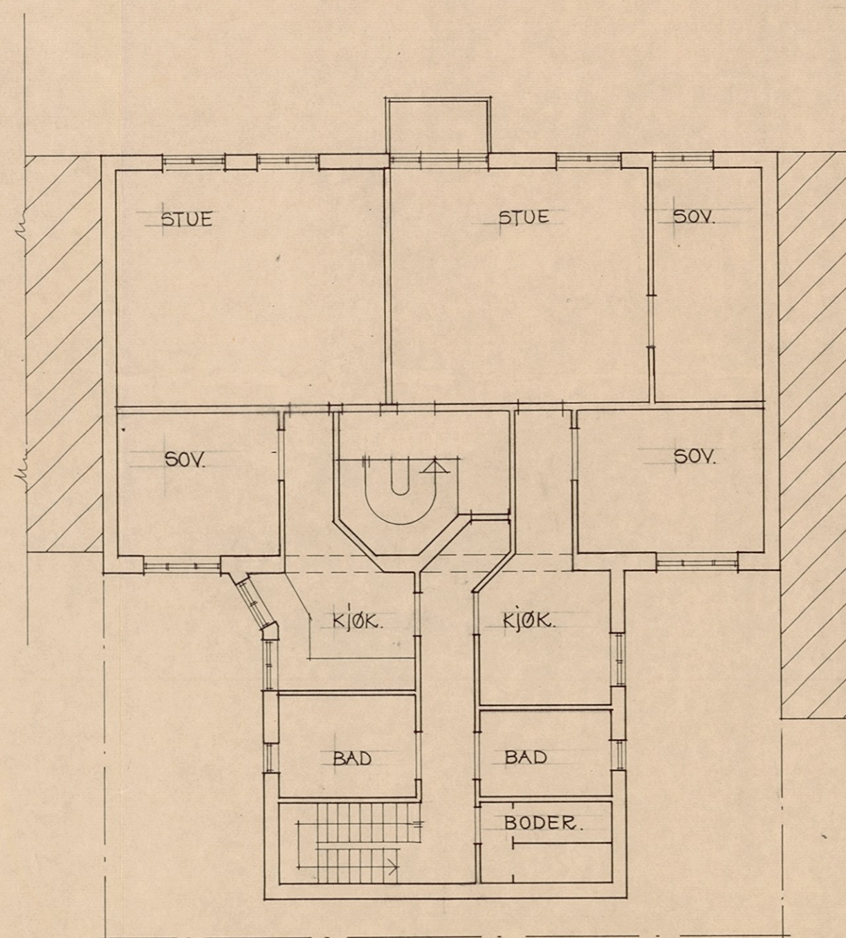
PLAN 2.ETASJE
