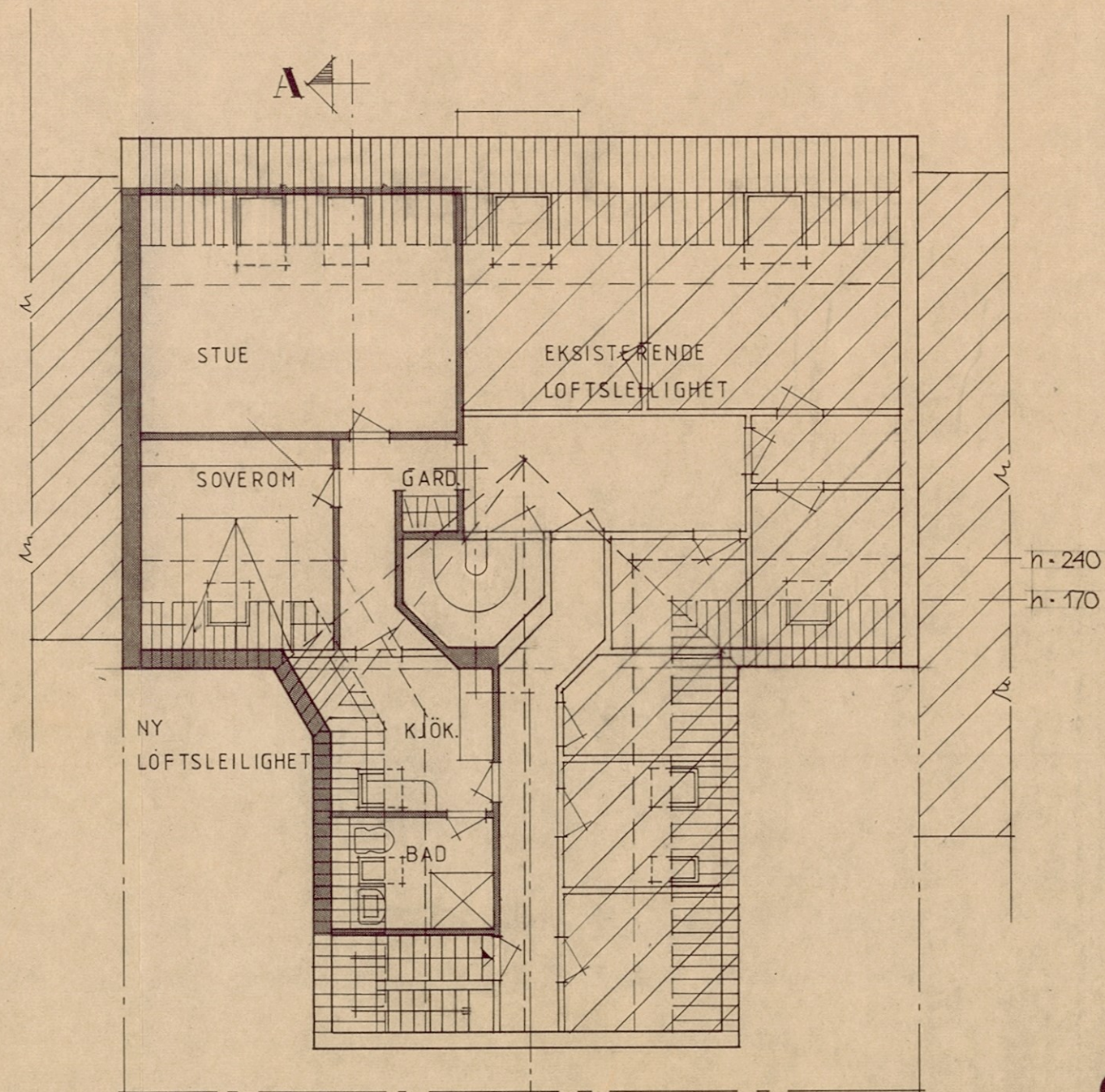
PLAN-LOFT — ENDRET
