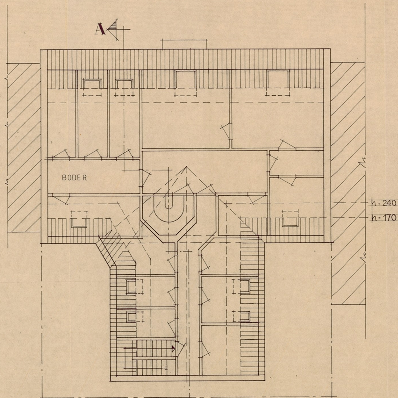
PLAN-LOFT — EKSISTERENDE
