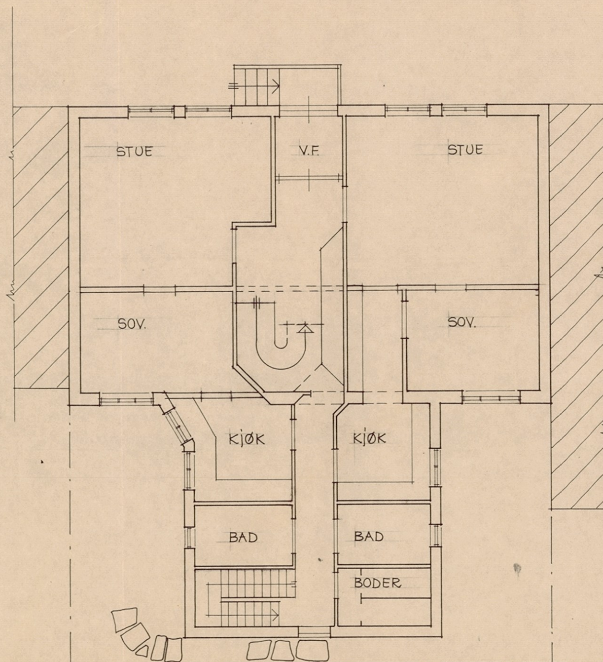
PLAN 1.ETASJE
