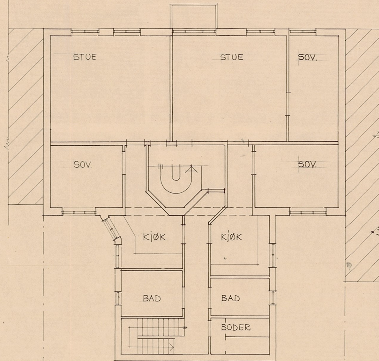
PLAN 3. ETASJE
