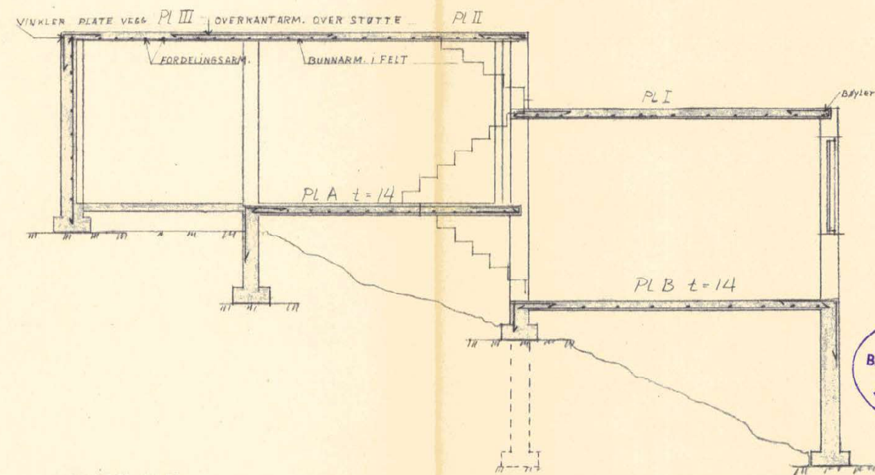
SNITT A-A
