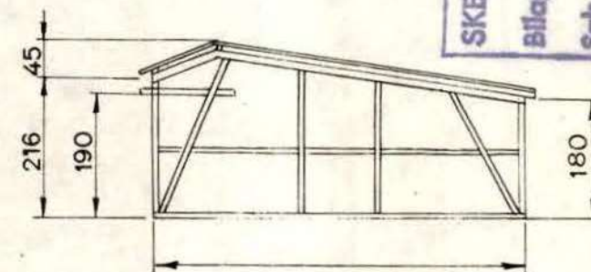
Snitt: A-A
