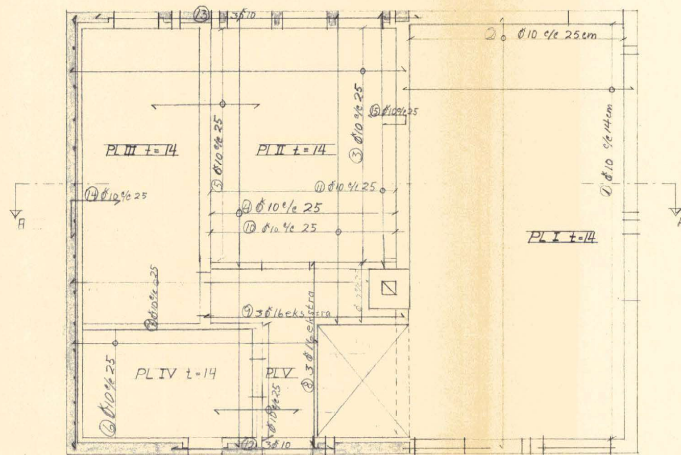
1. ETG. PLAN
