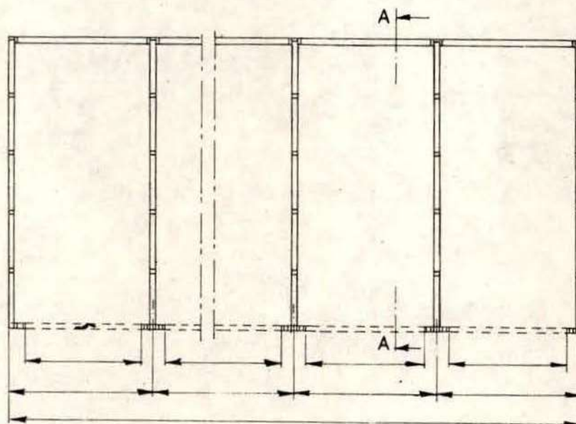
Plan Serie - garasje
