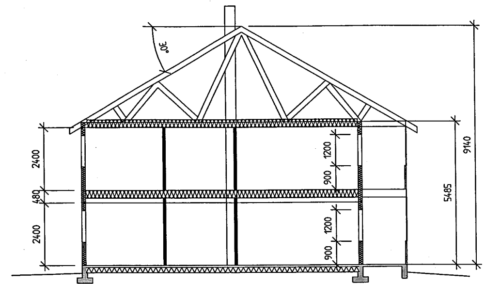
SNITT A-A
