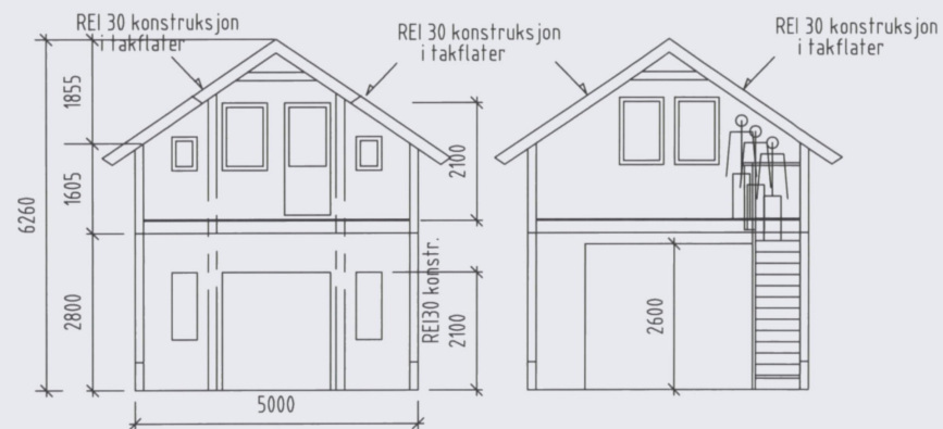
TYPISK SNITT FRITTLIGGANDE NAUST
