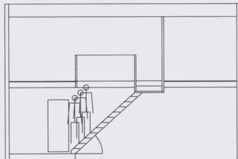
TYPISK LENGDESNITT FRITTLIGGANDE NAUST
