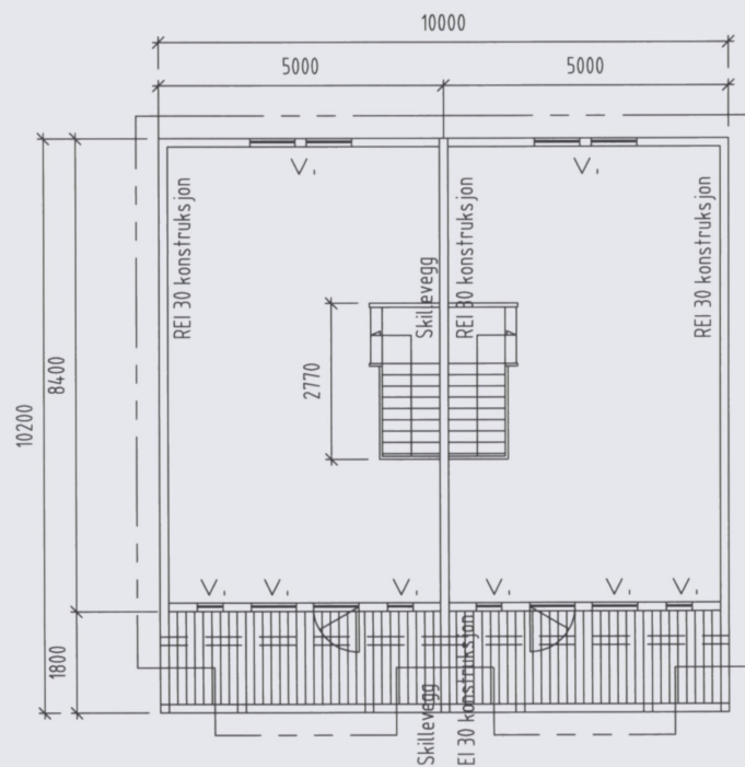
LOFTPLAN FRITTLIGGANDE NAUST
