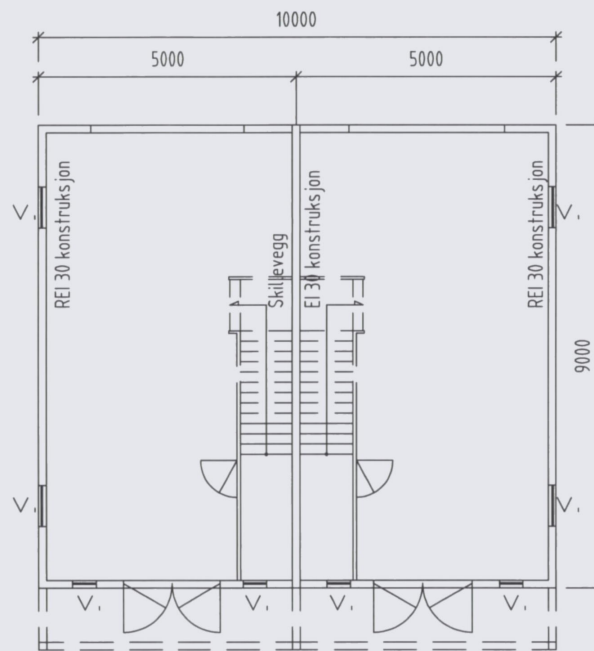
GRUNNPLAN FRITTLIGGANDE NAUST
