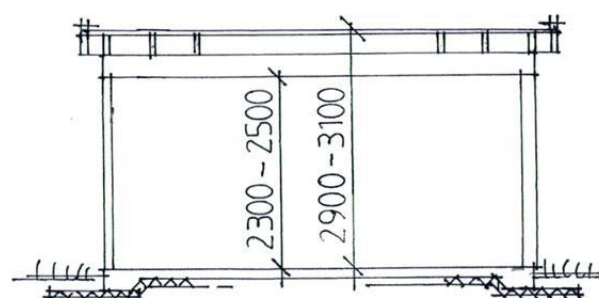
SNITT
