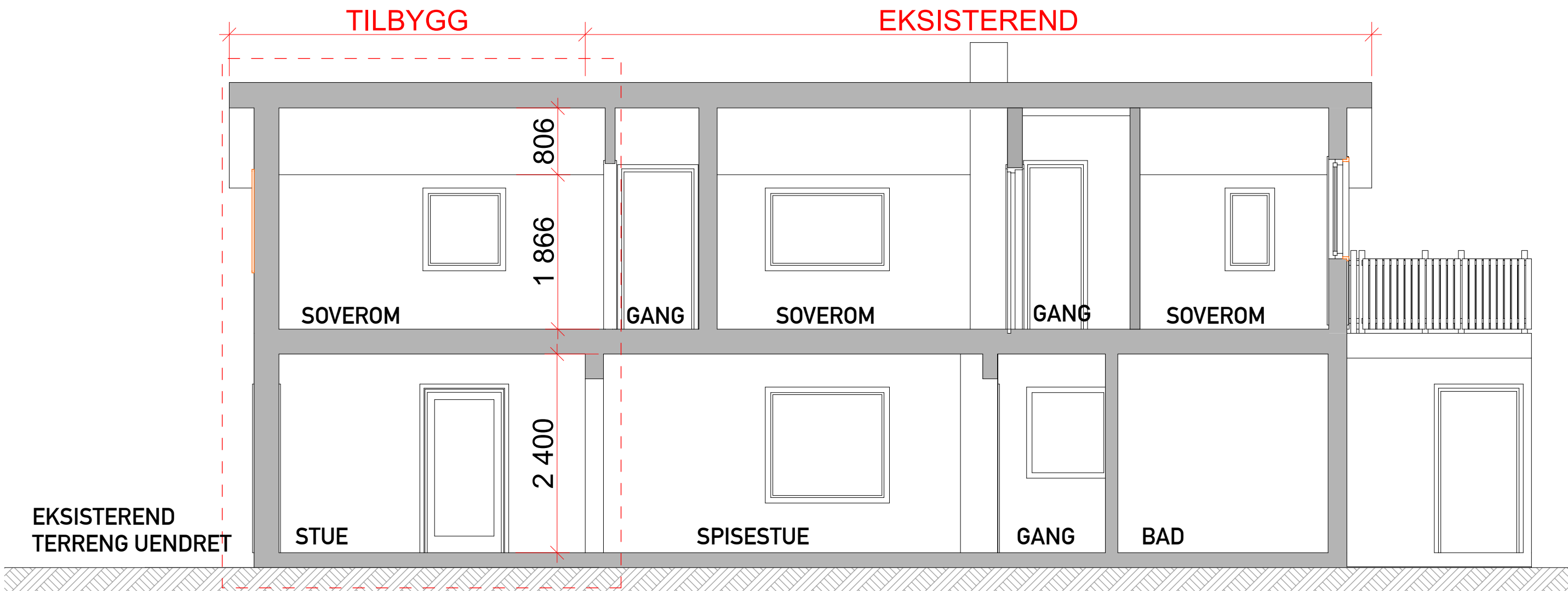
Snitt A
