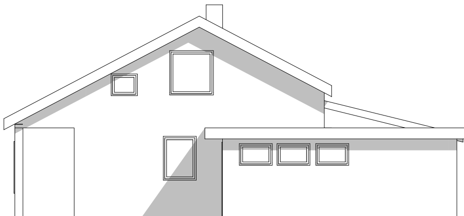
Fasade Øst 1:100
