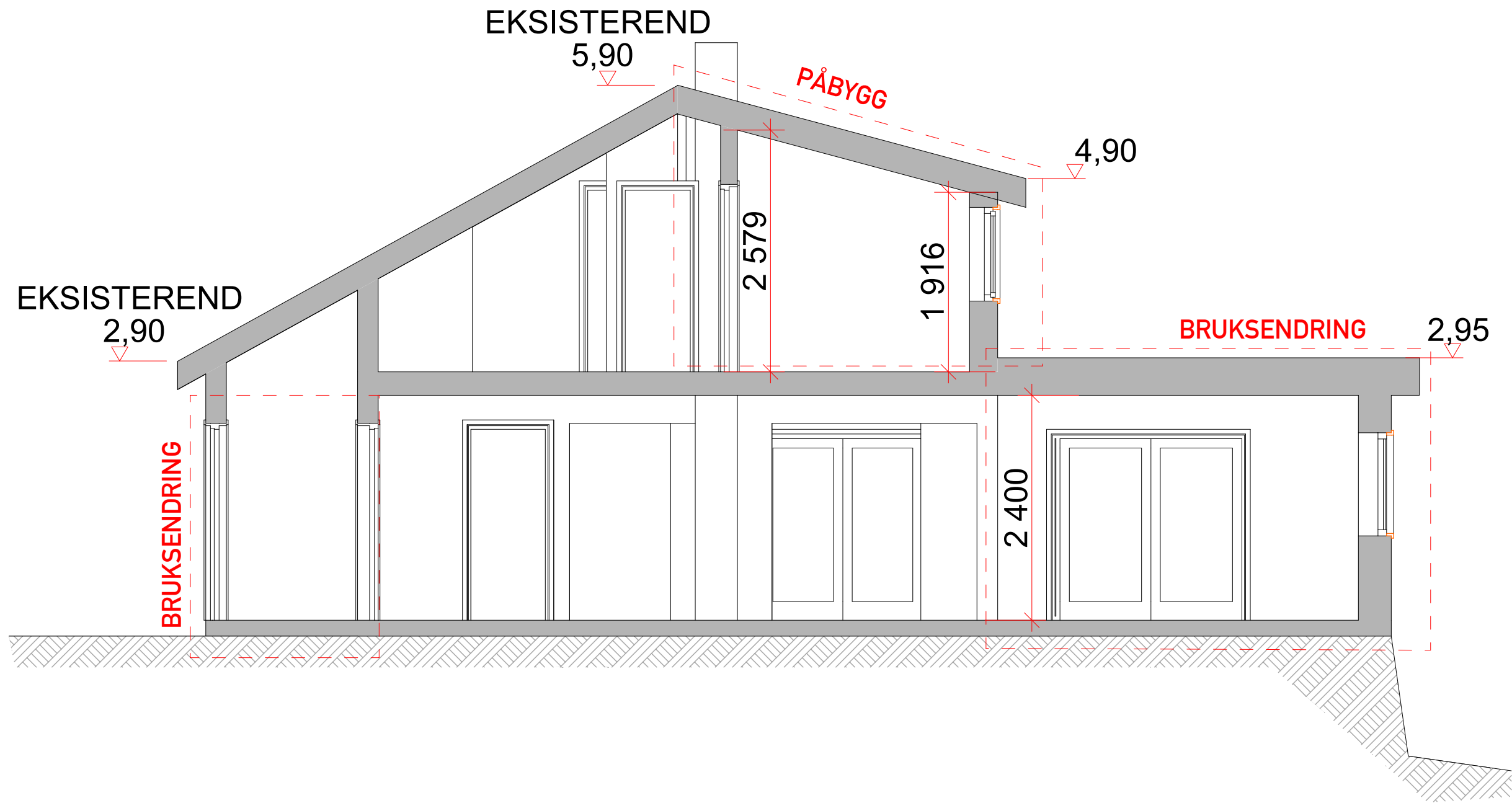
Snitt B
