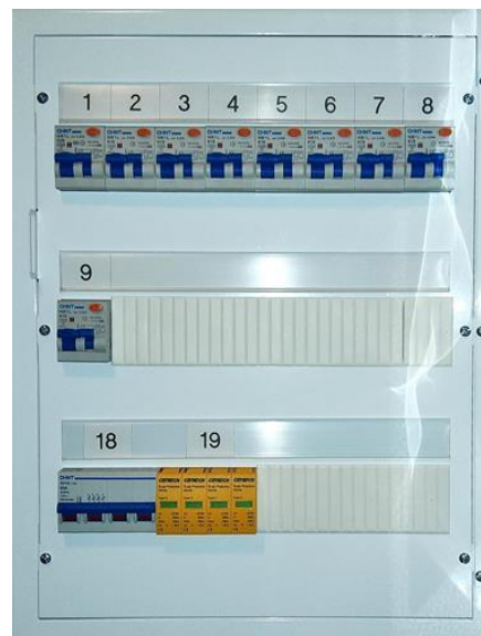
Forenklet vurdering av det elektriske anlegget - [Sikringsskap]
