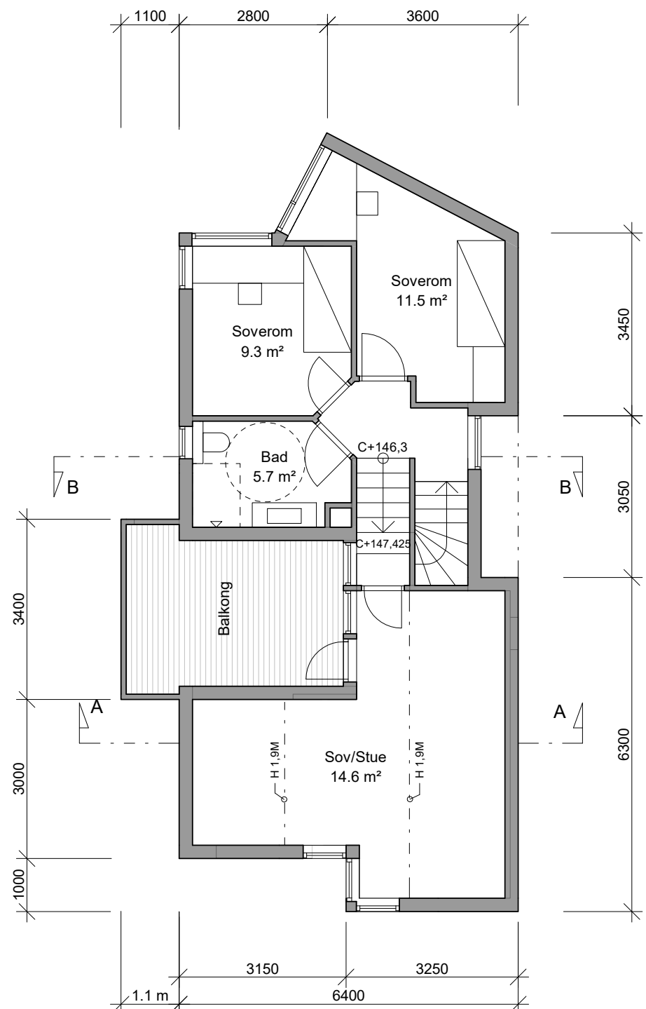
PLAN 2. ETASJE BRA= 51M 2
