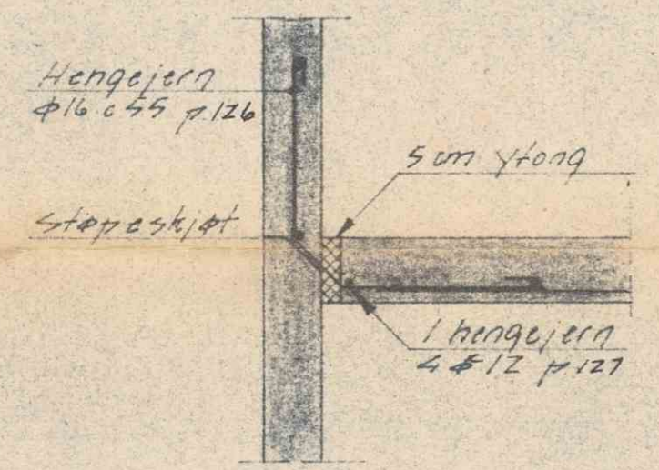
SNITT VED TRAPPEHUS M. 1/20
