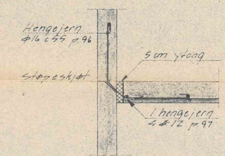
SNITT VED TRAPPEHUS M 1/20
