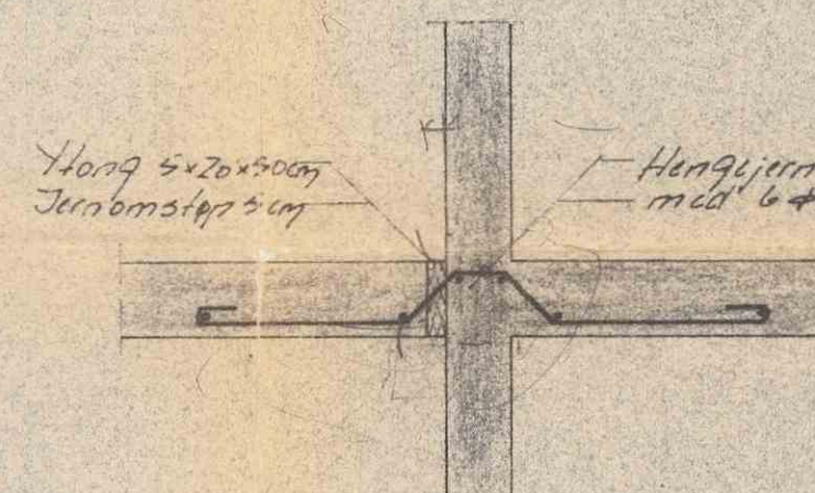
SNITT 3-3
