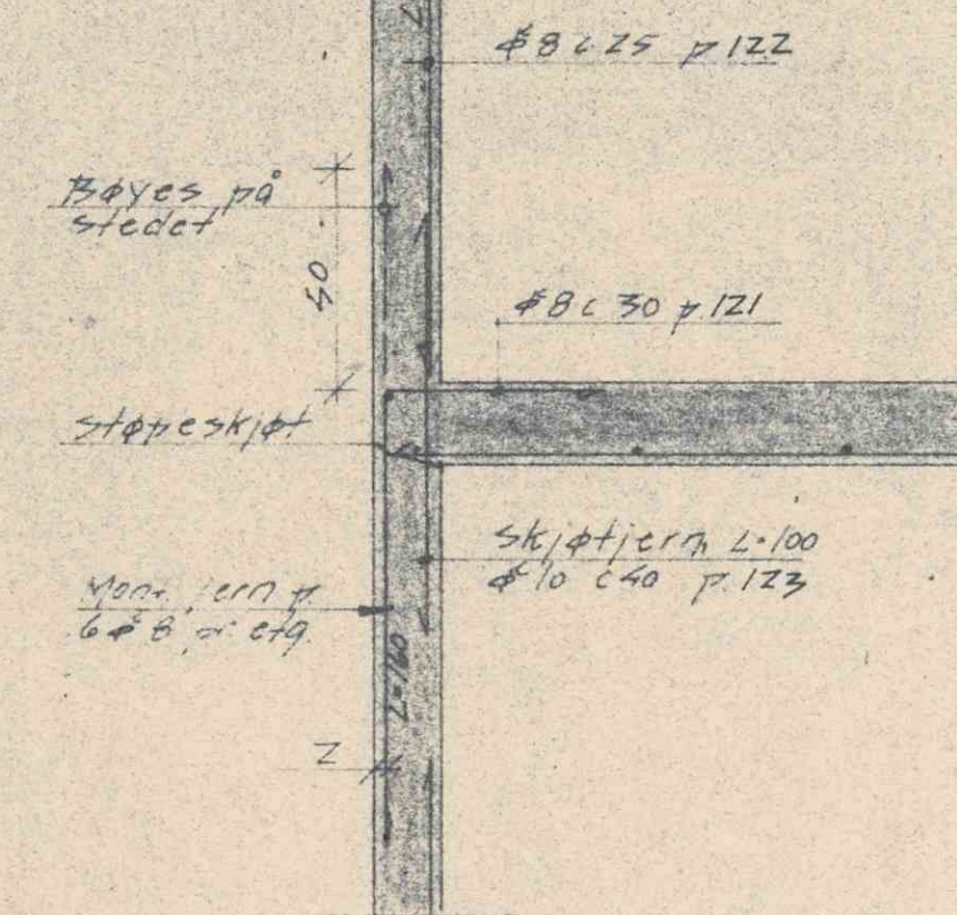
SNITT VED GAVL M. 1/20
