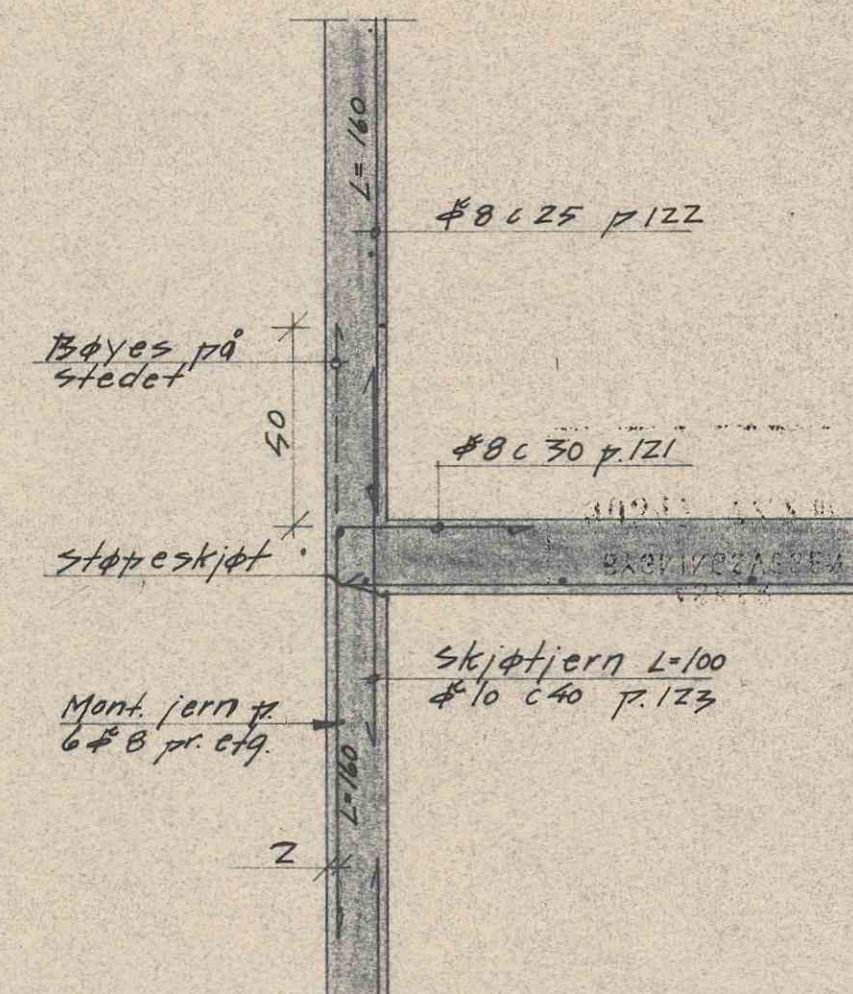
SNITT VED GAVL M: 1/20
