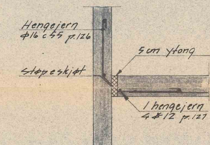
SNITT VED TRAPPEHUS M: 1/20
