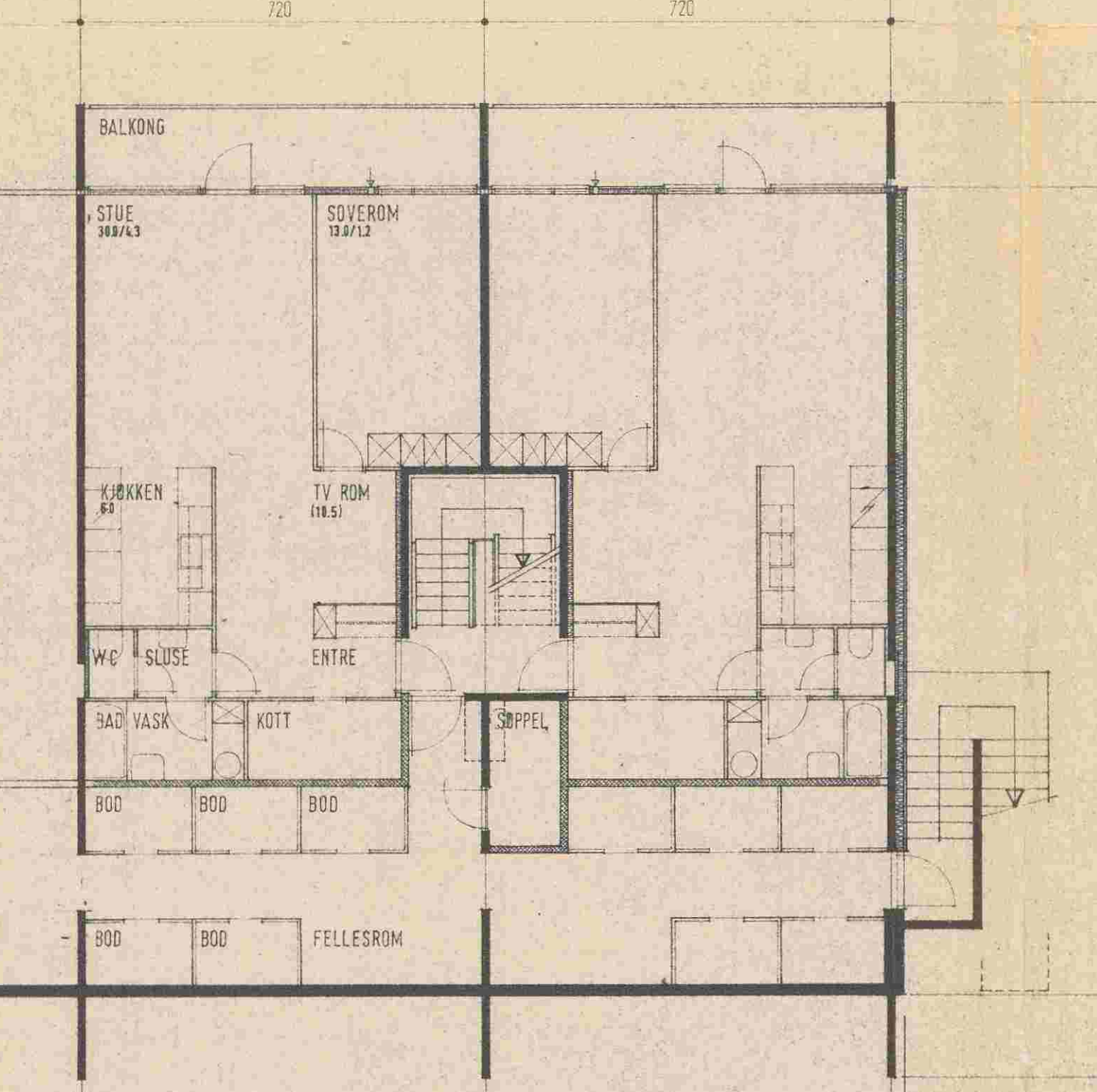
PLAN AV 2. U.ETG.
