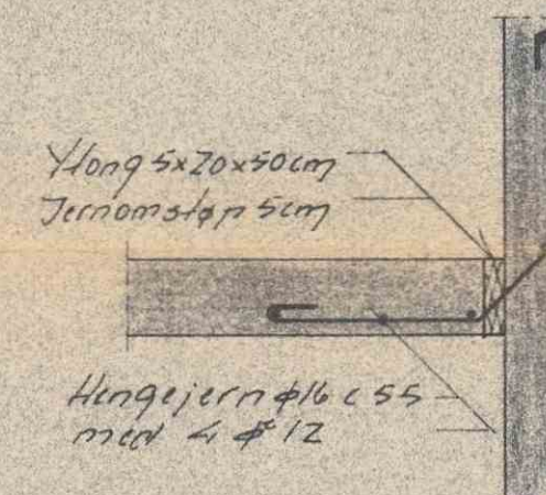
SNITT 4-4
