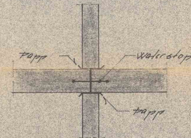
HORIZONTALSKITT BAKMUR.
