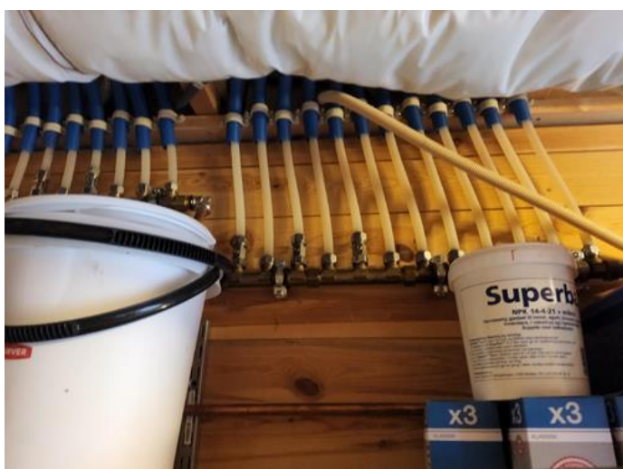
Vannrør (Sjekkpunkter utover det som er inkludert i andre rom) - [Fordelerstammer for rør-i-rør. ]
