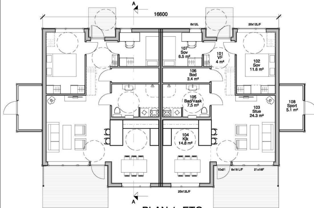
PLAN 1. ETG 1 : 100
