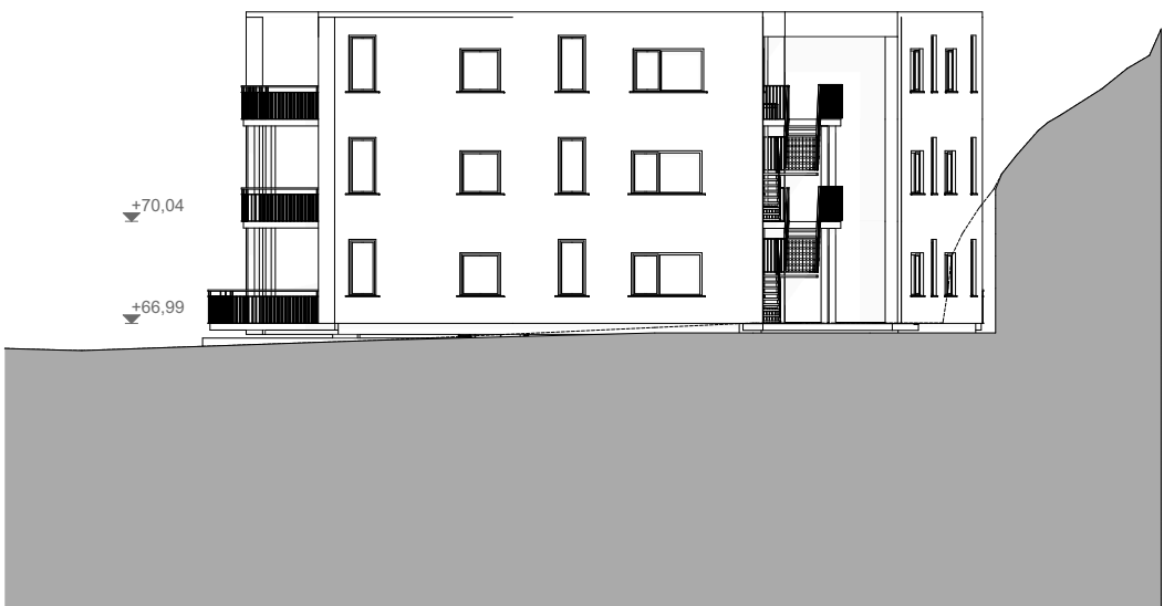
BB1 Fasade mot øst
