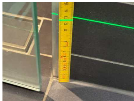
Fallforhold ca. 125 mm overkant gulv ved dusjsone
