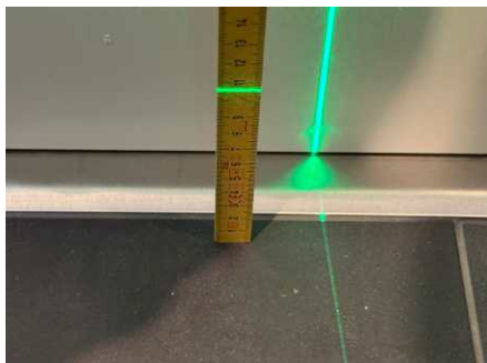
Fallforhold ca. 105 mm overkant gulv ved terskel
