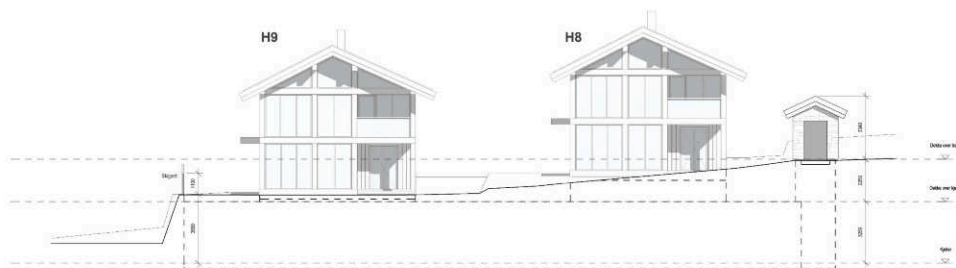
K-4001 - Oppriss nord
