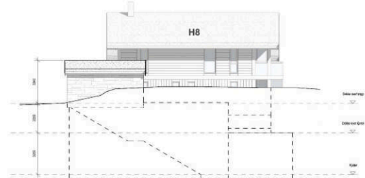
K-4001 - Oppriss vest
