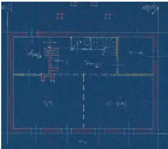
Eksisterende plantegning av kjeller
