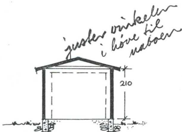
SNITT ENKEL
