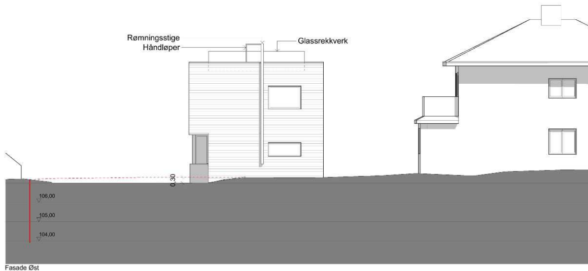
Fasade Øst
