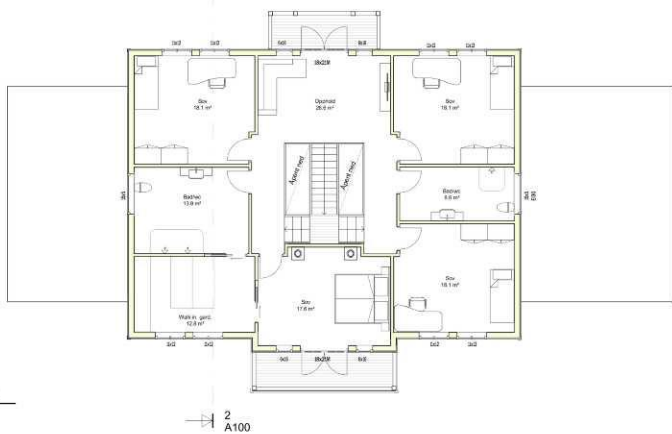
Plan 2 etg. 1 : 100
