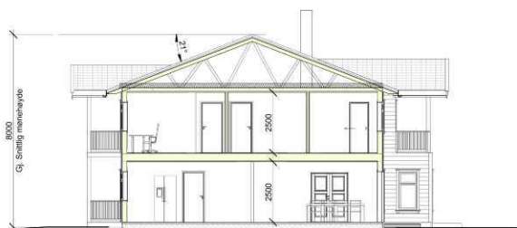
Snitt a-a 1 : 100
