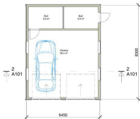
Plan 1 : 100
