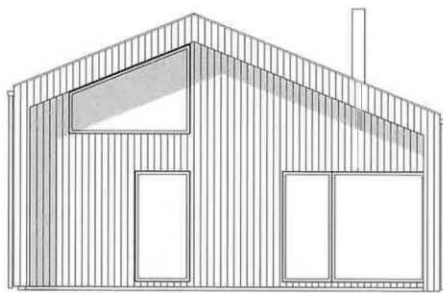
Fasade Sør
