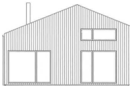
Fasade Nord
