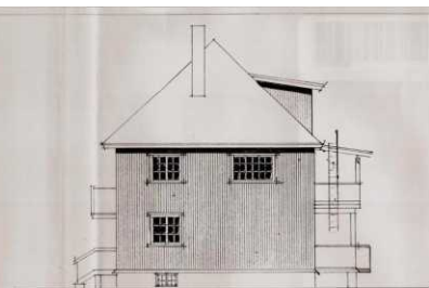
NÄRRENDEN FASAD
