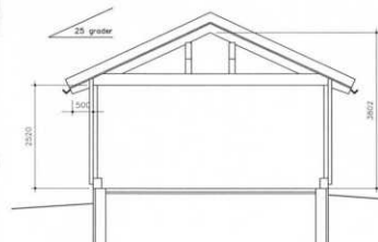
SNITT B-B
