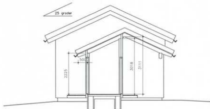
SNITT A-A
