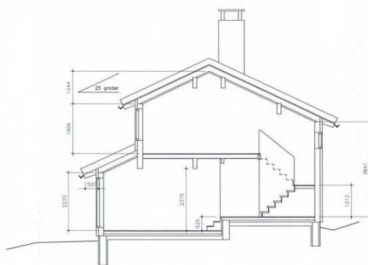
SNITT B-B
